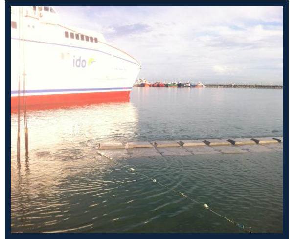
YENİKAPI – BANDIRMA FERİBOTLARI BLOK RIHTIM İNŞAATI İŞİ
