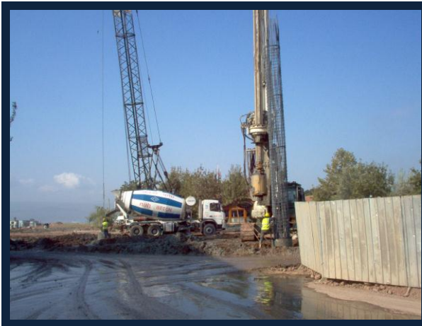
KOCAELİ BÜYÜKŞEHİR BELEDİYESİ -D100 KÖPRÜLER İNŞAATI FORE KAZIK UYGULAMASI -
