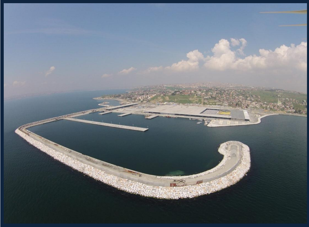
BEYLİKDÜZÜ / GÜRPINAR BALIKÇI BARINAKLARI İŞİ FİNAL FOTO - I
