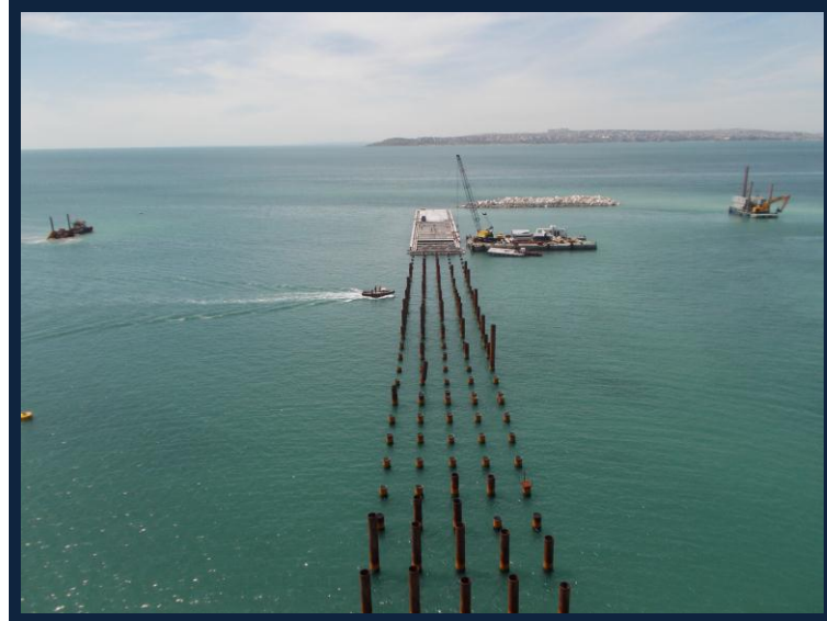
KAZIK ÇAKIMI – PREKAST KİRİŞ&DÖŞEME MONTAJI ve TOPPING BETONU UYGULAMASI
