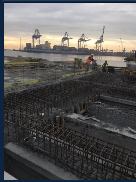
MARDAŞ – İSKELE YENİLEME / GÜÇLENDİRME PROJESİ - 2021
